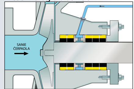
Obrázok 1 – všetky krúžky sú orientované na tesnosť
