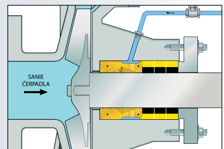
Obrázok 3 – Chesterton DualPac Superset™
